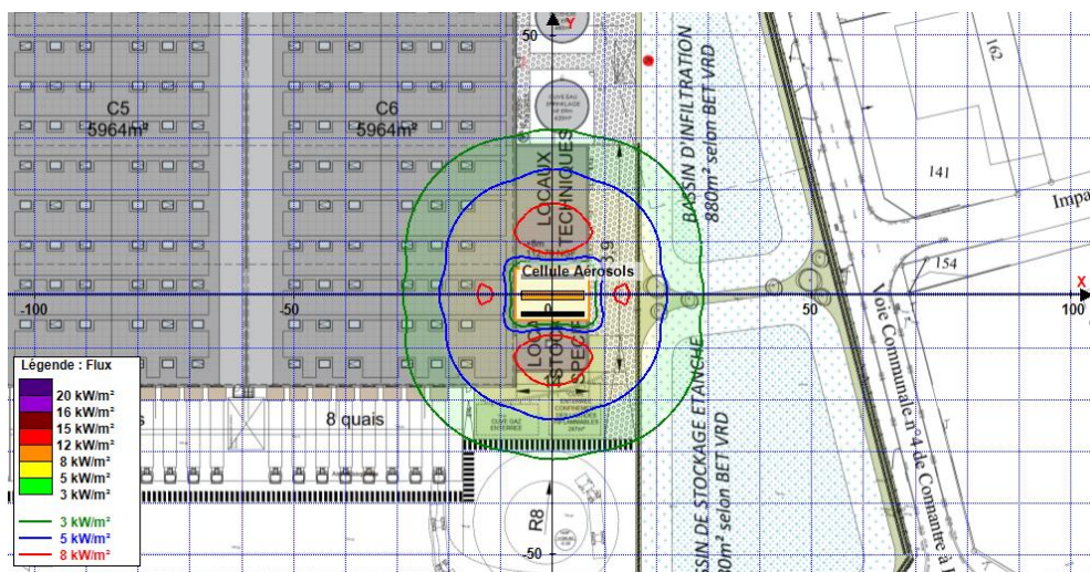
Illustration n° 14 : Modélisation FLUMILOG – Cartographie des effets thermiques – Cellule C6-A
