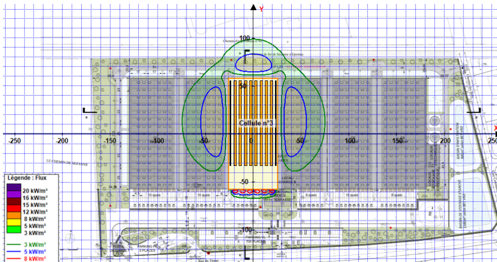
Illustration n° 9 : Modélisation FLUMILOG – Cartographie des effets thermiques – Cellule C4
